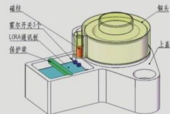
图1 阀头结构图
